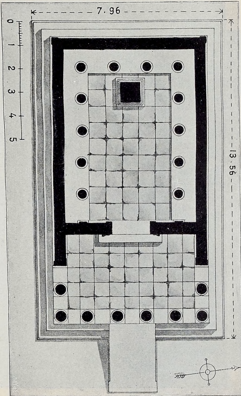
Εικ. 15. Κάτοψις ναού Ἀφροδίτης (ἀναπαράστασις).
