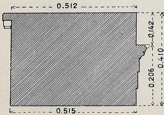
Είχ. 5 Τομή γωνιακοῦ ἐπιστυλίου τῆς βορειοδυτικῆς ἢ νοτιοδυτικῆς γωνίας τοῦ τοίχου.
