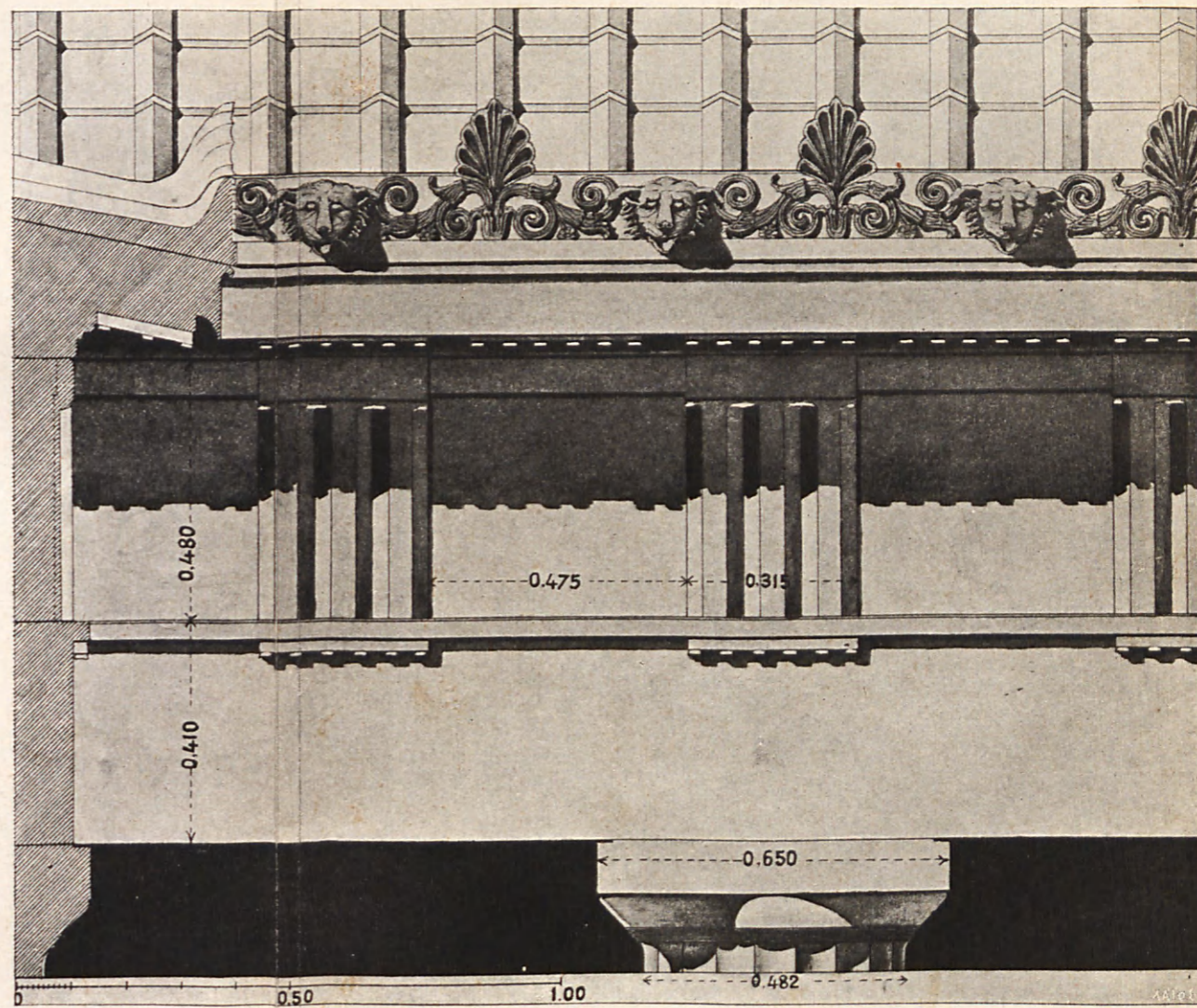
Εἰκὼν 2. Θριγκὸς ναοῦ Ἀρτέμιδος.
