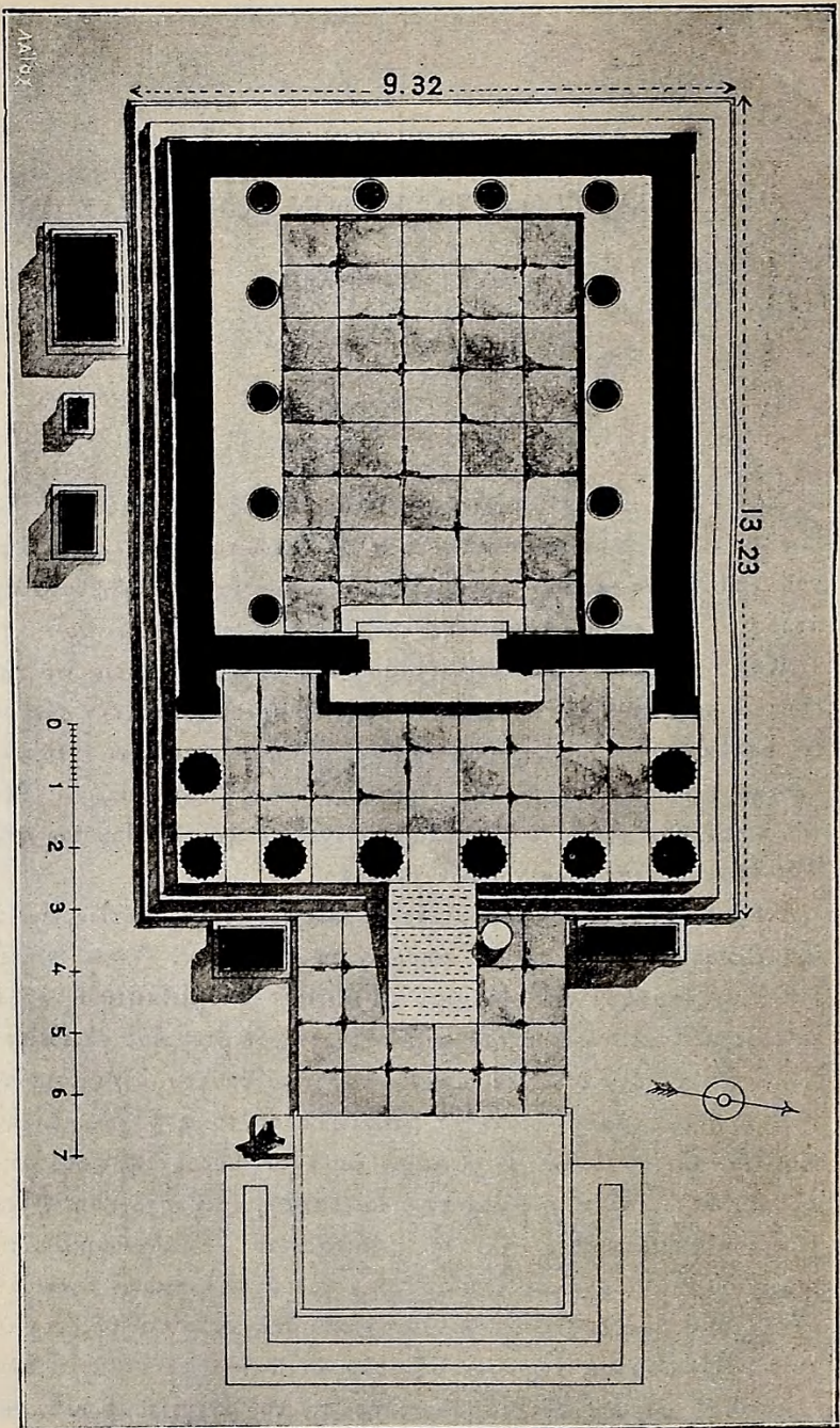
Ειχ. 1. Κάτοψις τοῦ ναοῦ τῆς Ἀρτέμιδος (ἀναπαράστασις).
