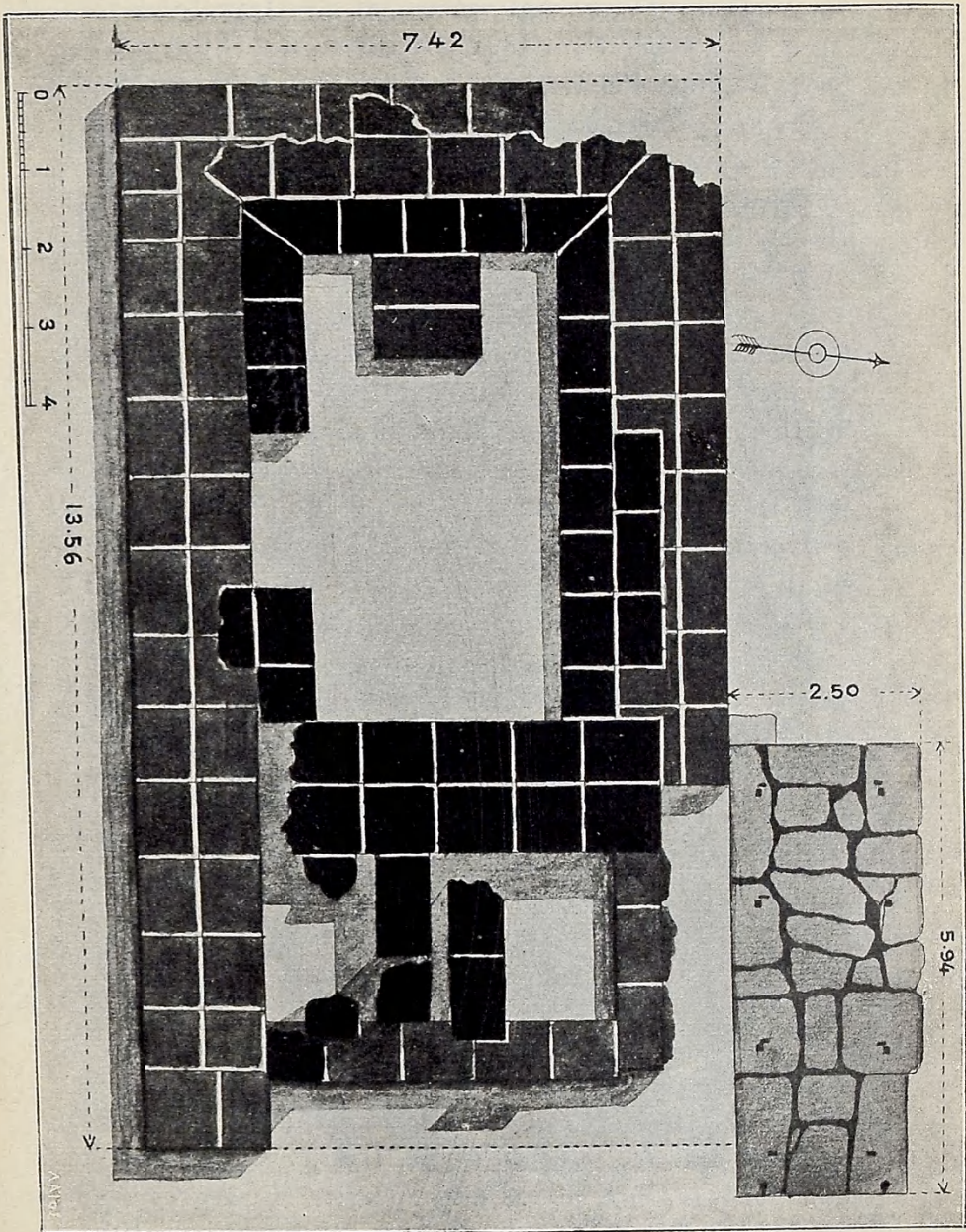
Fig. 11. Καπίδωμα ναού Θιμίου.
