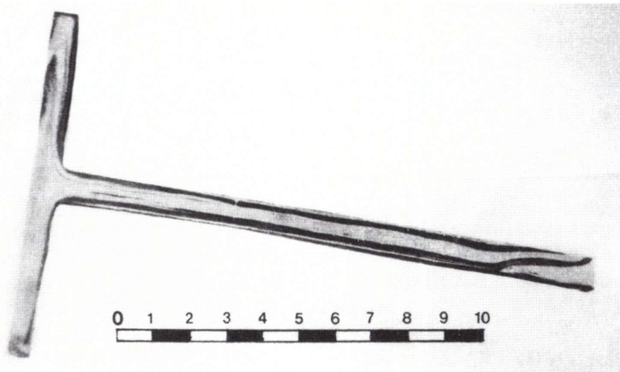
Είκ. 7. Μακροσκοπική εξέταση ενός συνδέσμου μετά τη λείανση, στίλβωση και προσβολή με Nital 10%. Έμφανίζεται η μακροσκοπική δομή του σιδερένιου ταύ, όπου μία μαλακή σιδερένια στρώση έχει συγκολληθεί ανάμεσα σε δύο σκοτεινόχρωμες χαλύβδινες στρώσεις με σφρηλασία σε θερμοκρασία περίπου 1250°C - 1300°C.
