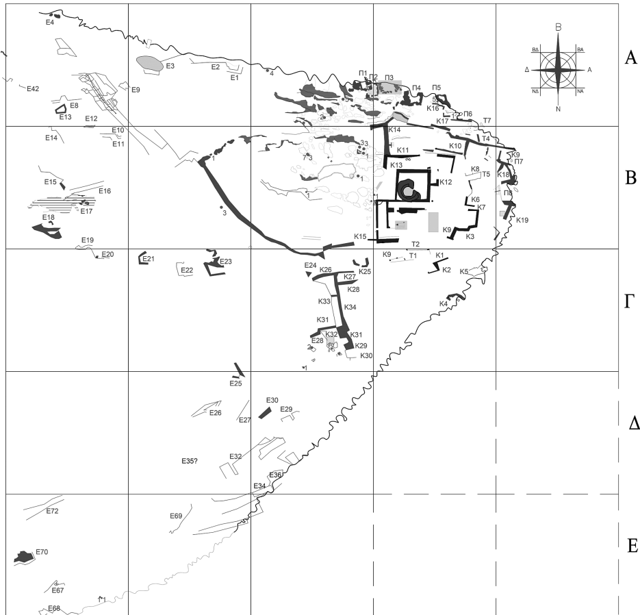
15. Βαθὺ Ἀστυπалаίας. Γενικὸ τοπογραφικὸ σχέδιο.
