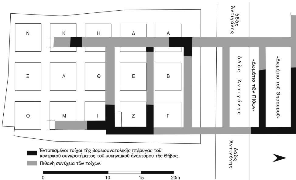
10. Θήβα. Γενικὸ τοπογραφικὸ τῆς ἀνασκαφῆς.
