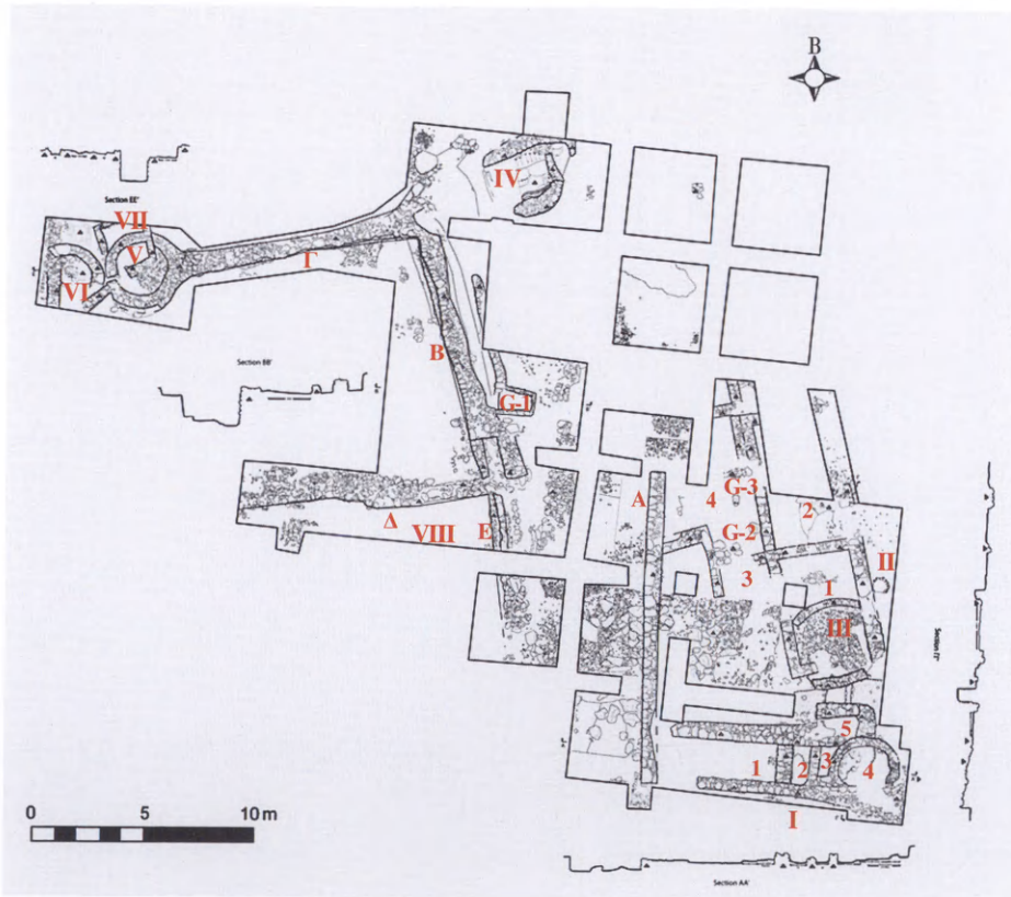
7 Μυκῆνες. Κάτω Πόλη, κάτοψη τῆς ἀνασκαφῆς.
