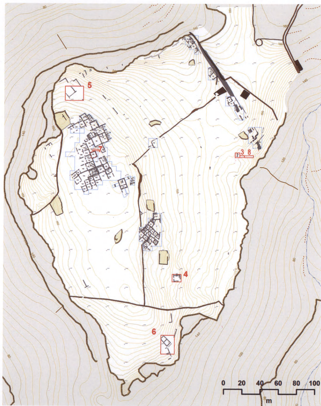
43 Ζαγορά Άνδρου. Τοπογραφικό σχέδιο με τις θέσεις τῶν ἀνασκαφικῶν τομῶν.
