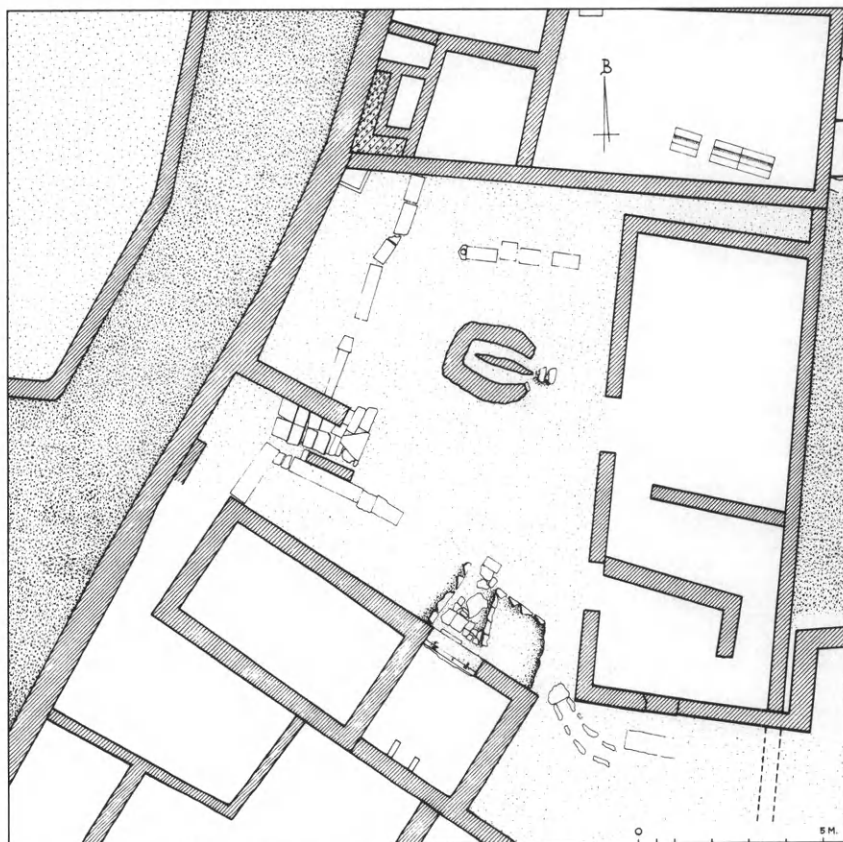
3 Πλατεία στη ΝΑ συνοικία του φρουρίου. Στο μέσον μεταλλευτικός κλίβανος· πίσω του θεμέλια πρόχειρης στοᾶς· κάτω στο μέσον, μικρὸς ναός.
