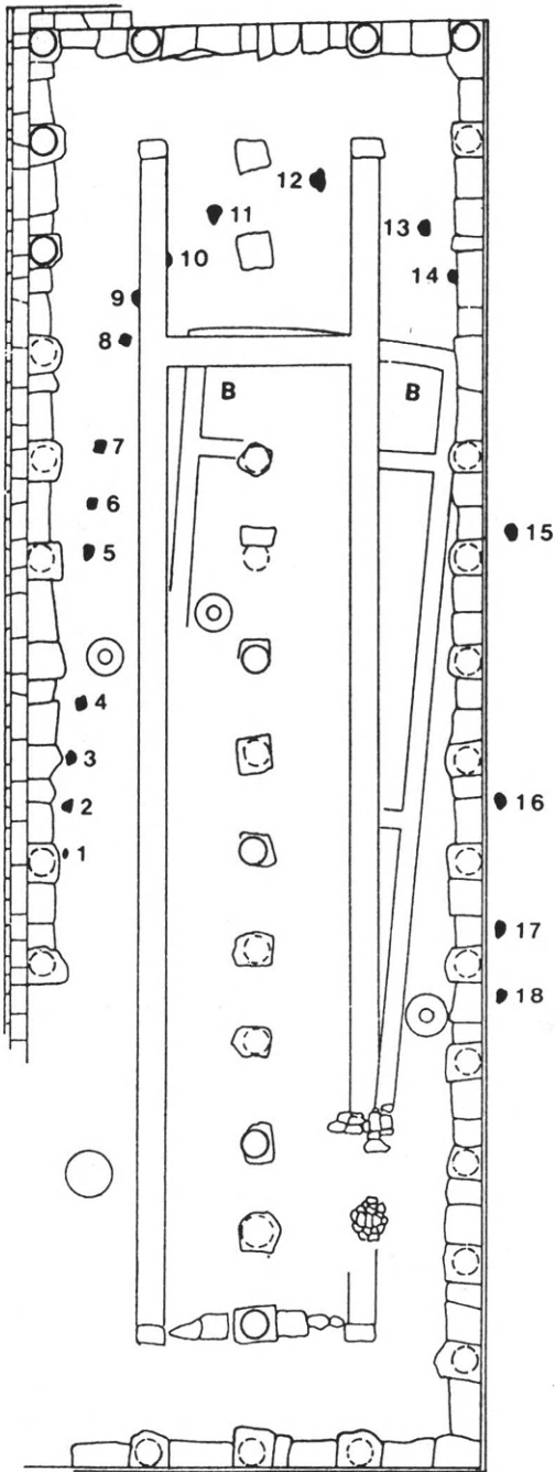
20 Τὸ σχέδιο τοῦ ναοῦ καὶ τοῦ μεγάρου Β μετὰ τὰς πλάκες τῆς “ἑλλειπτικῆς περιστασης” κατὰ τὸν Ρωμαῖο.
