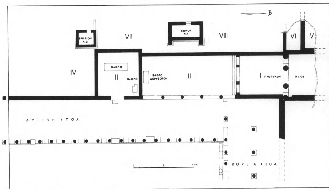
17 Κάτοψη τοῦ Γυμνασίου.
