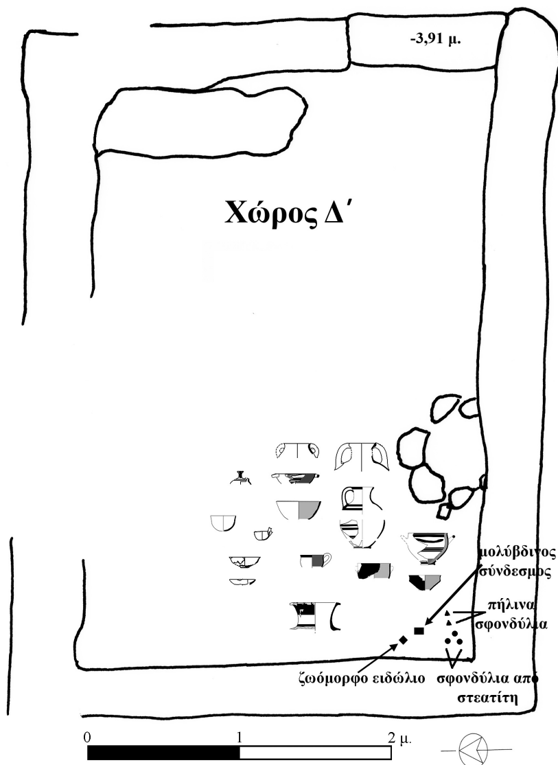
Σχ. 2. Τὸ δάπεδο τοῦ χώρου Δ' με τὸν ἐλάχιστο ἀριθμὸ ἀγγείων καὶ μικροεπιτημάτων ποὺ βρίσκονταν κατὰ χώραν.
