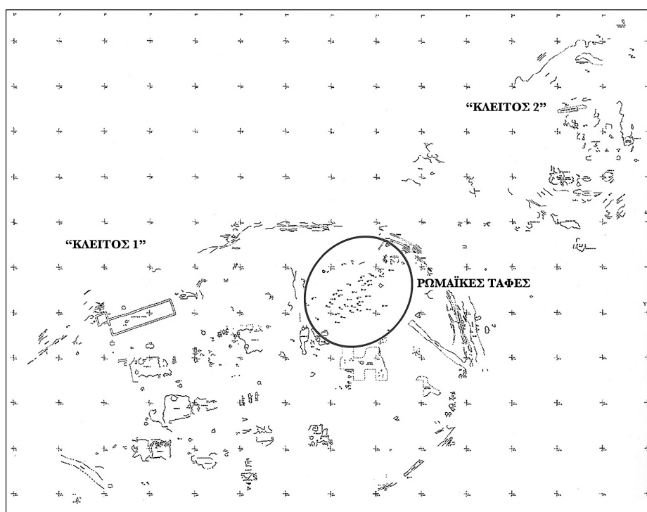
Είχ. 2. Τοπογραφικό σχέδιο του Κλείτου με σημειωμένους τους Κλείτο I και Κλείτο II.
