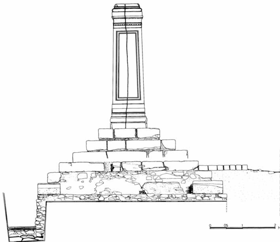
Εἰκ. 7. Ἡ βόρεια ὄψη τοῦ βάθρου τοῦ κίονα μετὰ τὴν ὑποδομὴν του (τομὴ τοῦ ἀνασκαφικοῦ σκάμματος ἀπὸ Α. πρὸς Δ.) (σχέδ. τῆς ΙΣΤ΄ ΕΠΚΑ).
