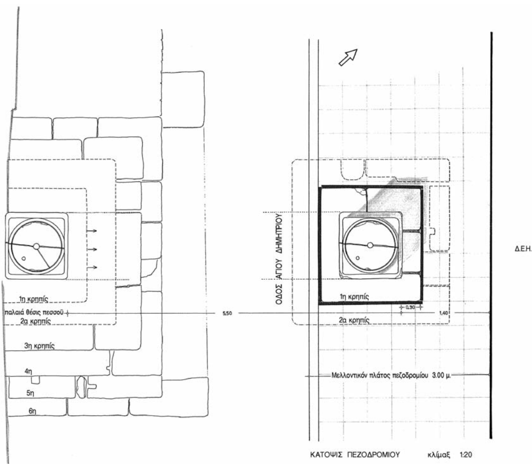
Εικ. 10. Κάτοψη του βάθρου του κίονα α) άριστερά in situ, πριν από τη μετακίνησή του και β) δεξιά στη νέα του θέση στο πεζοδρόμιο της οδού (σχέδ. της ΙΣΤ' ΕΠΚΑ).
