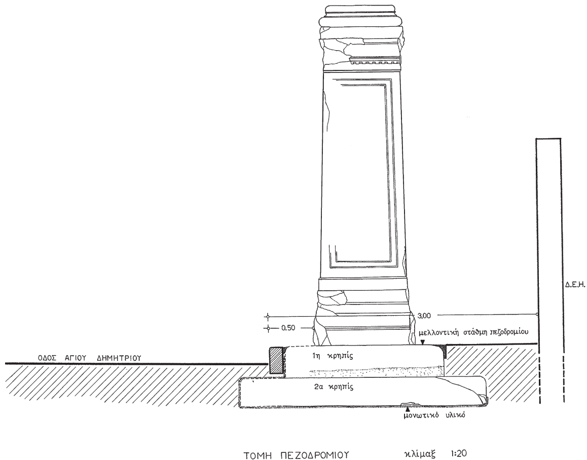
Εἰκ. 11. Ἡ ἀνατολική ὄψη τοῦ βάθρου τοῦ κίονα μετὰ τὶς δύο ἀνώτερες βαθμίδες τῆς κρηπίδας, ὅπως τοποθετήθηκε μπροστὰ στὸν τοῖχο τοῦ ὑποσταθμοῦ τῆς ΔΕΗ (σχέδ. τῆς ΙΣΤ' ΕΠΚΑ).
