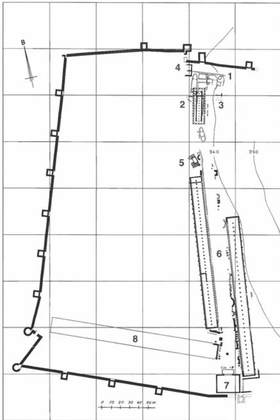
Είκ. 7. Τοπογραφικό σχεδιάγραμμα του ἱεροῦ καὶ τῆς ἀγορᾶς τοῦ Θέρμον. 1. ΥΕ οἰκισμός, 2. Ναὸς Ἀπόλλωνος καὶ Μέγαρον Β, 3. Ναὸς Λυσείου Ἀπόλλωνος, 4. Ναὸς Ἀρτέμιδος (;), 5. Κρήνη, 6. Πλατεία ἀγορᾶς μὲ τὶς στοές, 7. «Βουλευτήριον», 8. Νότια στοά.
