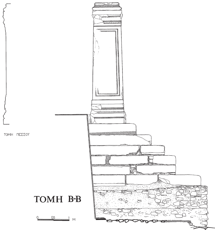
Εἰκ. 8. Ἡ ἀνατολική ὄψη τοῦ βάθρου τοῦ κίονα μετὰ τὴν ὑποδομὴ του (τομὴ τοῦ ἀνασκαφικοῦ σκάμματος ἀπὸ Ν. πρὸς Β.) (σχέδ. τῆς ΙΣΤ' ΕΠΚΑ).
