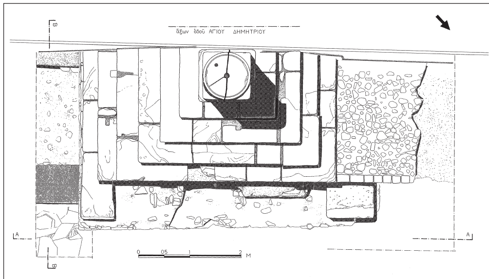
Εἰκ. 6. Κάτοψη τοῦ βάθρου τοῦ κίονα, ὅπως εἶχε διατηρηθεῖ in situ (σχέδ. τῆς ΙΣΤ΄ ΕΠΚΑ).
