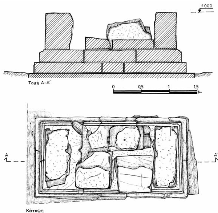
11α-β. Σχέδιο κάτοψης και τομής του «βάθρου της Αιτωλίας» (διαστ. άνω επιφάνειας βάθρου: 2,35×1,10).
