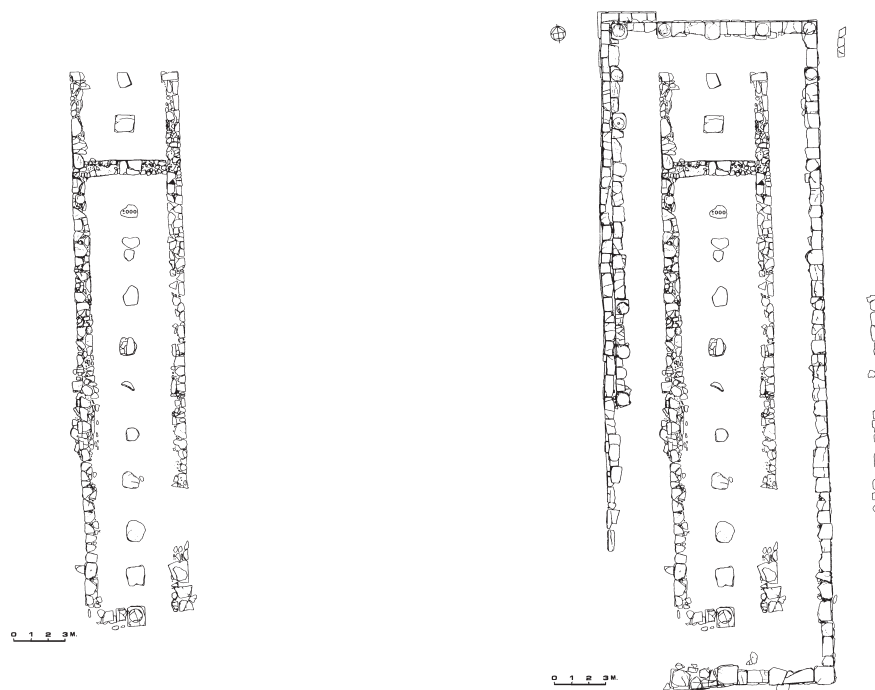
Εἰκ. 5. α. Ὁ πρῶτος ναὸς τοῦ Ἀπόλλωνος, σηκὸς μὲ μεσαία κιονοστοιχία καὶ ἴσως ὀπισθόδομο, τελευταῖο τέταρτο 7ου αἰ. π.Χ. β. Ὁ ναὸς τοῦ Ἀπόλλωνος μετὰ ἀπὸ τὴν προσθήκη περιστυλίου, τέλος 3ου - ἀρχὲς 2ου αἰ. π.Χ.
