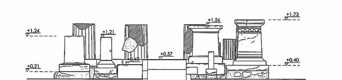
Σχ. 1. Σχεδιαγράφημα της πρόσοψης του ναού του Άσκληπιού και της Ύγείας.
