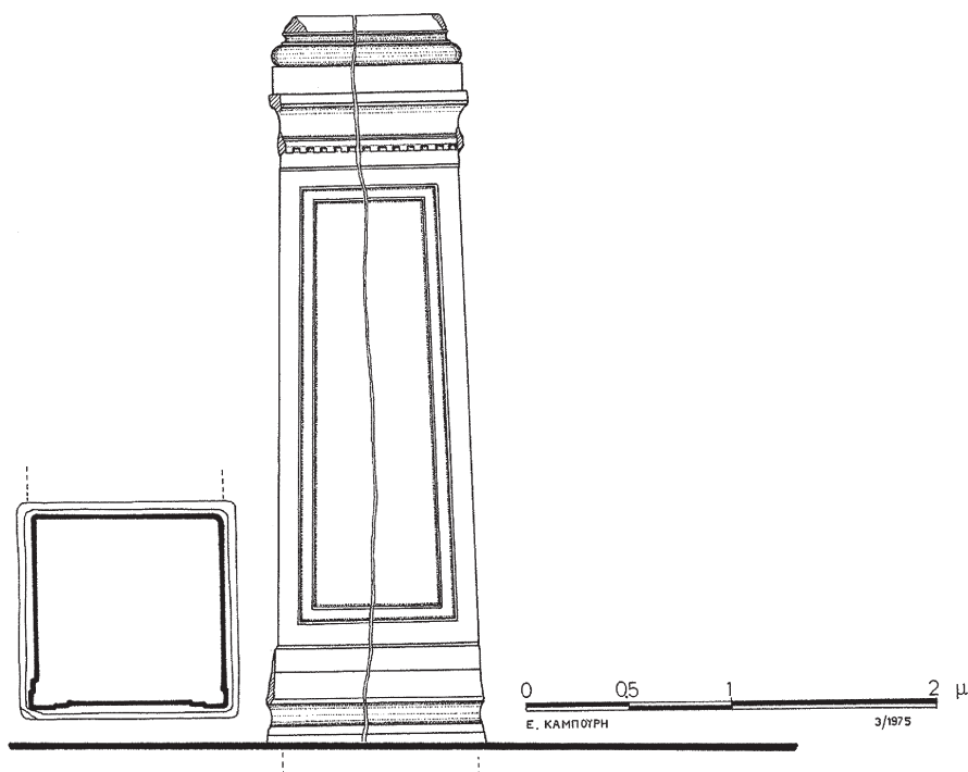
Εἰκ. 14. Ὁριζόντια τομὴ καὶ βόρεια ὄψη τοῦ βάθρου τοῦ κίονα (σχέδ. τῆς ΙΣΤ' ΕΠΚΑ).
