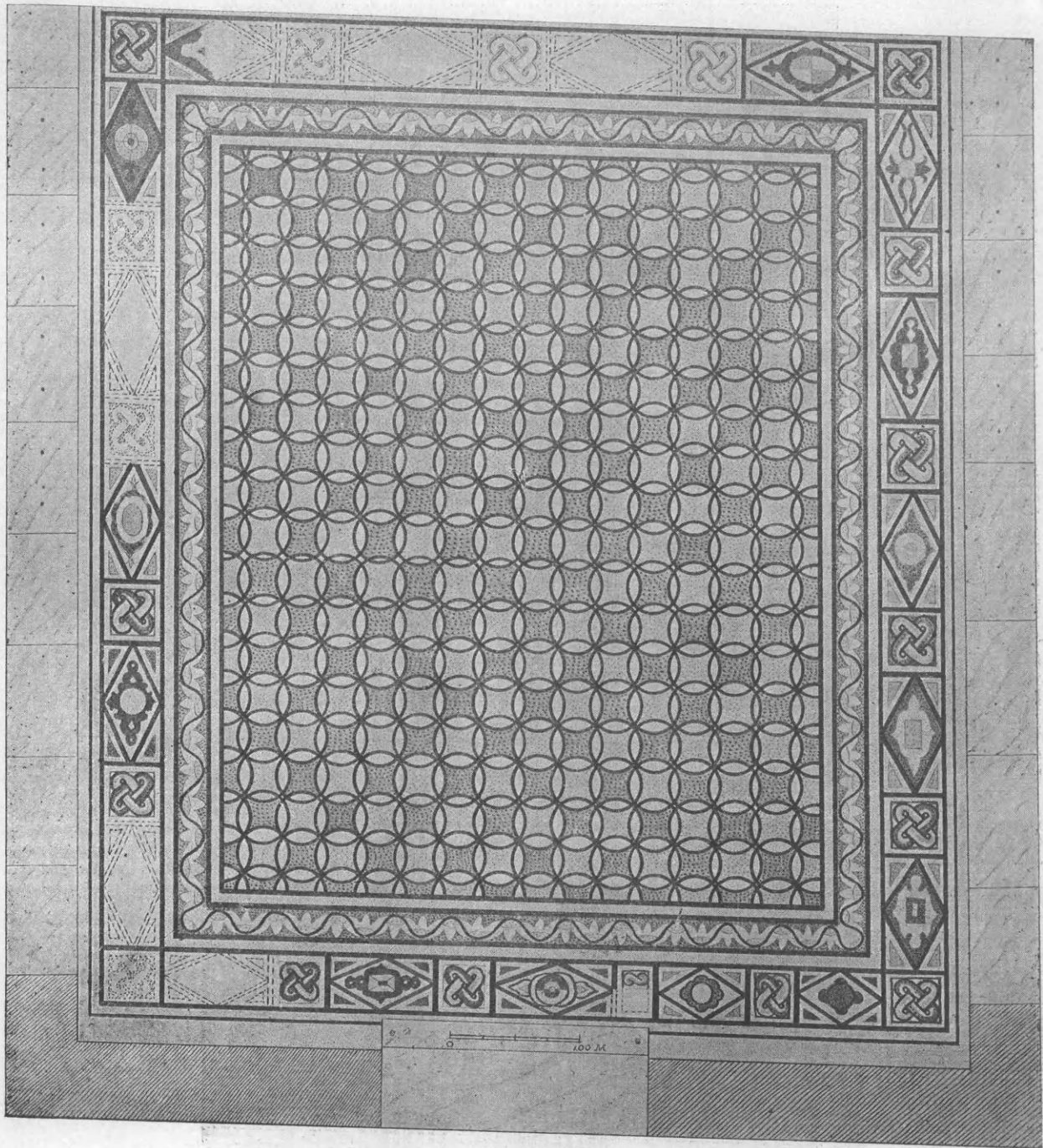
Εἰκ. 24. α' τμήμα μουσειωτοῦ ἐδάφους (εἰκ. 13 καὶ 14, μ), Μῆκος 7,95, πλάτος 6,95.
