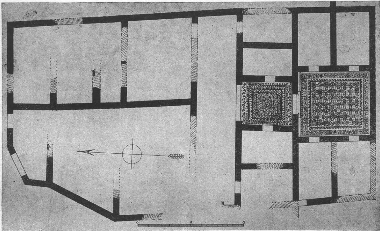
Εἰκ. 32. Οἰκοδόμημα μετὰ μωσαϊκῶν (ἴδε εἰκ. 33 καὶ 34 καὶ εἰκ. 35).
