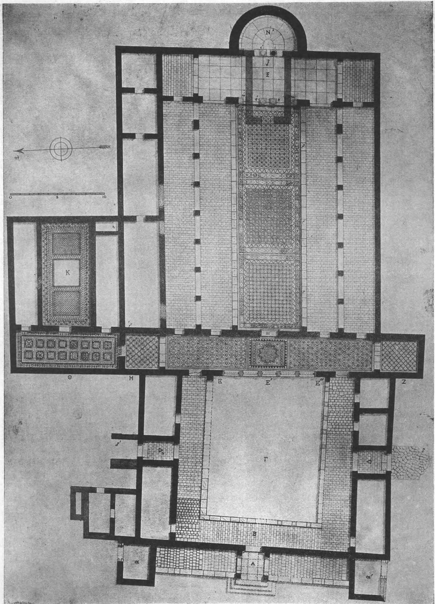
Εἰκ. 13. Ἀψιδωτὸν μετὰ μωσαϊκῶν οἰκοδόμημα δυνάμενον νὰ ἐκληφθῆ ὡς Ἀγορὰ μετὰ Βασιλικῆς. Ἴδε καὶ εἰκ. 15
