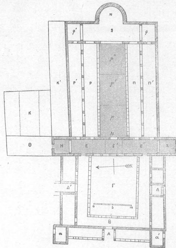
Εἰκ. 14. Τὸ ἐν εἰκ. 13 οἰκοδόμημα ἐμφανιζόμενον ὡς συμμετρικόν (δεδηλωμένον διὰ παχειῶν γραμμῶν). Διὰ τῆς προσθήκης τοῦ διὰ λεπτῶν γραμμῶν δεδηλωμένου κτίσματος γίνεται τὸ ὅλον οἰκοδόμημα ἄσύμμετρον.
