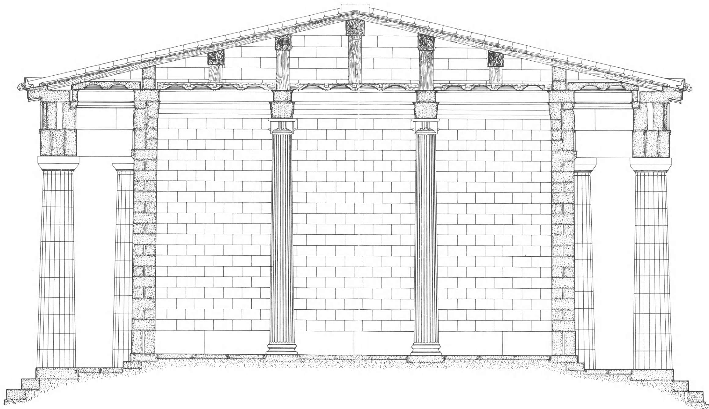
ΤΟΜΗ ΚΑΤΑ ΠΛΑΤΟΣ ΕΙΣ ΤΟΝ ΟΠΙΞΘΟΔΟΜΟΝ
