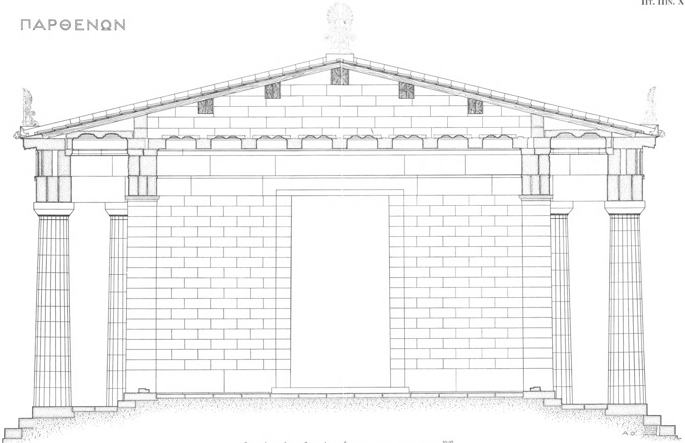
ΤΟΜΗ ΚΑΤΑ ΠΛΑΤΟΣ ΕΙΣ ΤΟΝ ΟΠΙΞΘΟΝΑΟΝ
