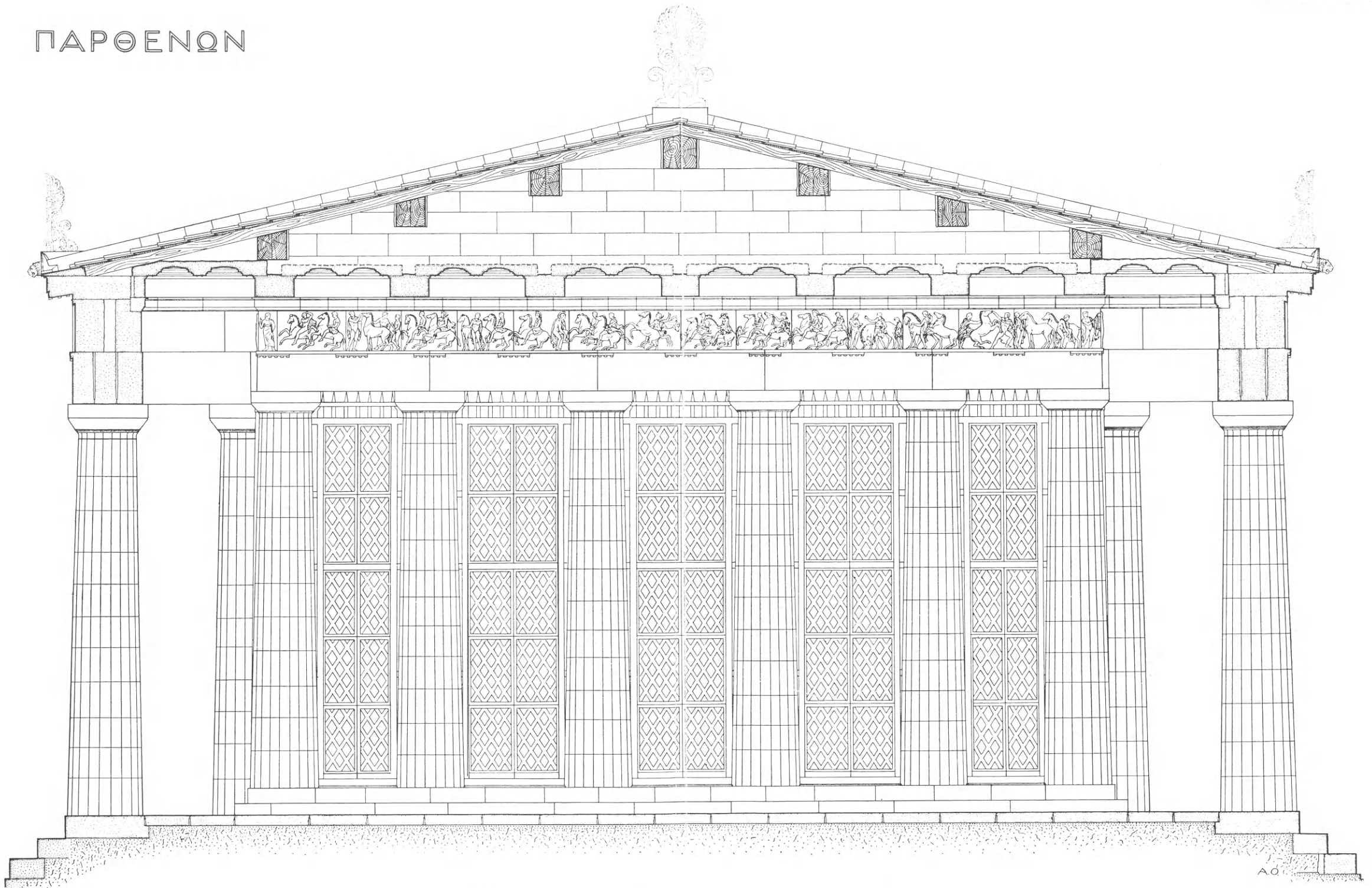
ΤΟΜΗ ΚΑΤΑ ΠΛΑΤΟΣ ΕΙΣ ΤΟ ΔΥΤ. ΠΕΡΙΣΤΥΛΙΟΝ
