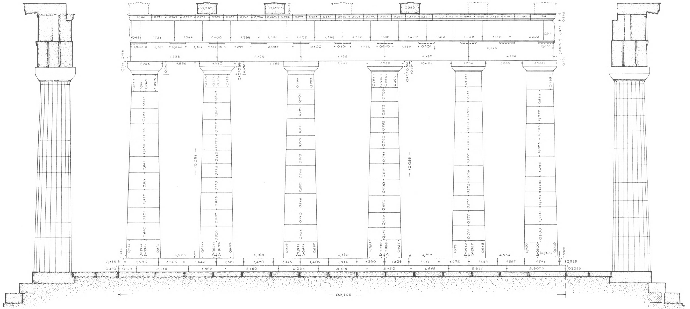
ΜΕΤΡΗΣΕΙΣ ΕΙΣ ΤΟΝ ΟΠΙΣΘΟΝΑΟΝ
