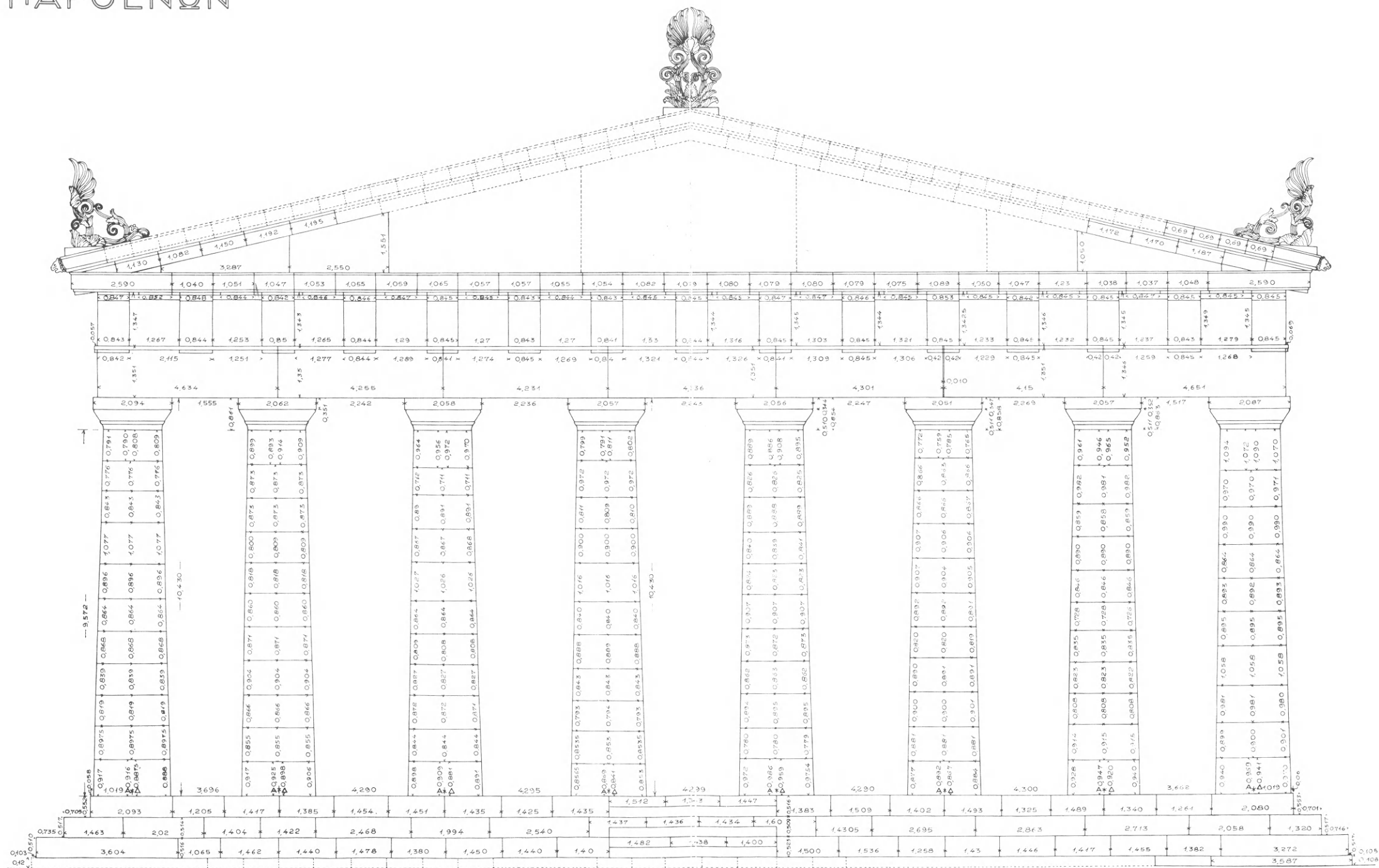
ΜΕΤΡΗΣΕΙΣ ΑΝΑΤΟΛΙΚΗΣ ΟΥΡΟΣ 1950-52
