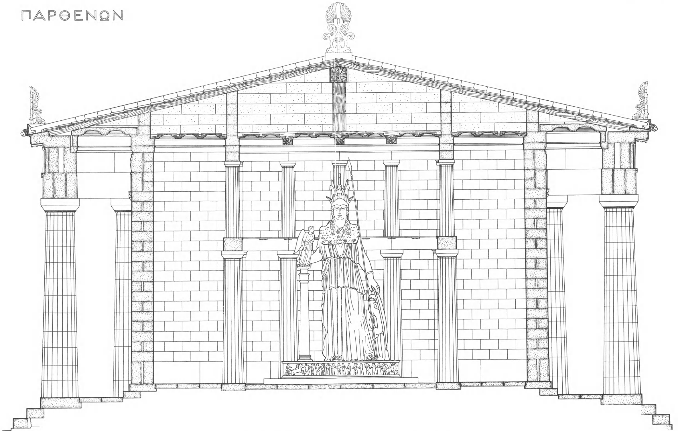
ΤΟΜΗ ΚΑΤΑ ΠΛΑΤΟΣ ΕΙΣ ΤΟΝ ΚΥΡΙΟΣ ΝΑΟΝ
