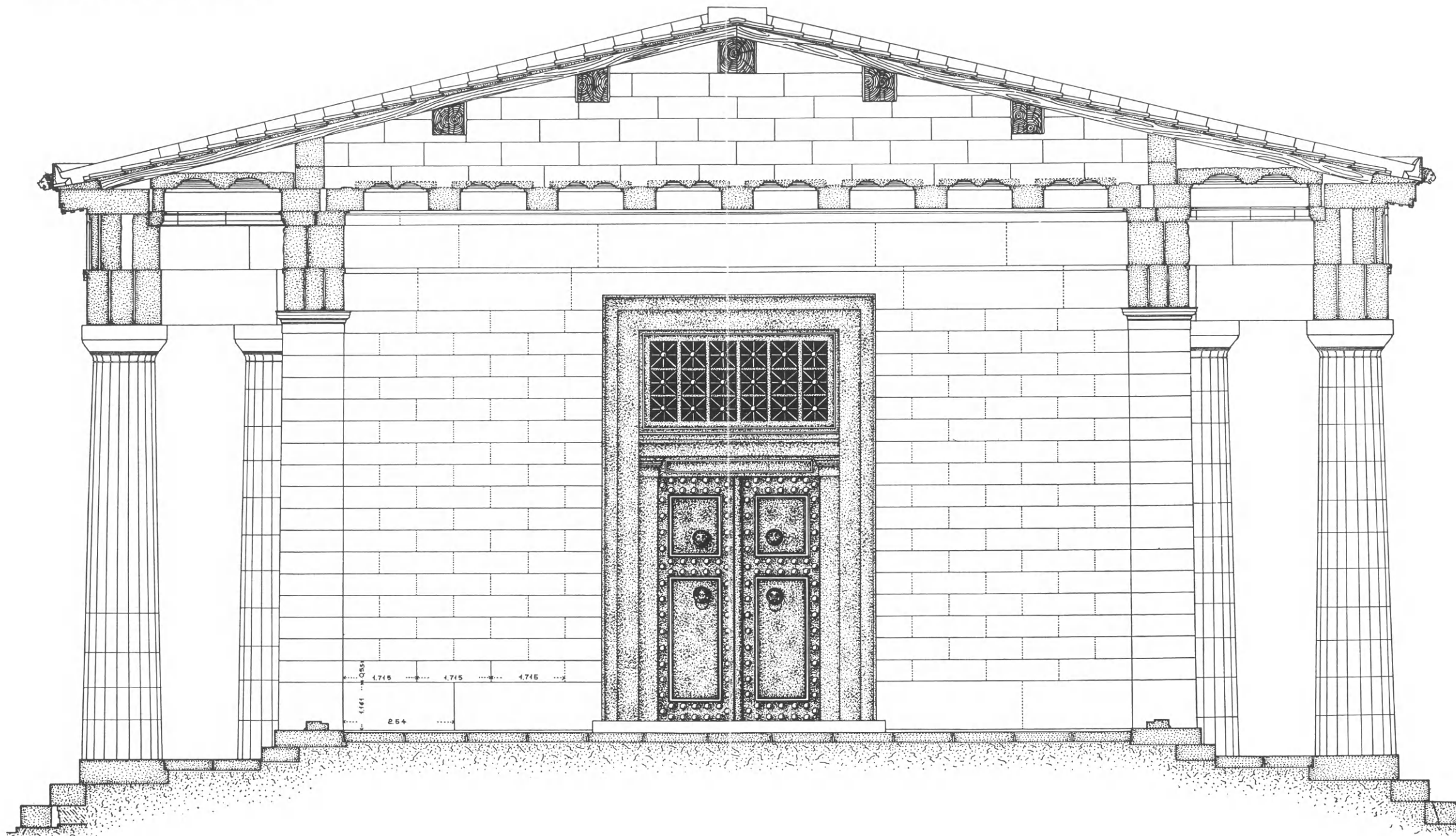
ΤΟΜΗ ΚΑΤΑ ΠΛΑΤΟΣ ΕΙΣ ΤΟΝ ΠΡΟΝΑΟΝ
