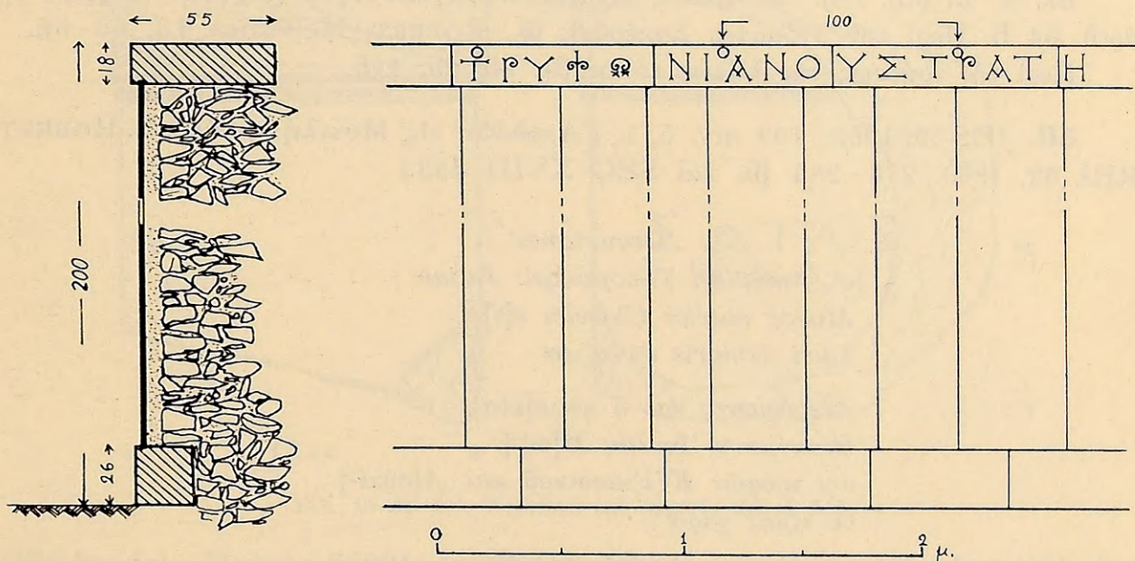
Εἰκ. 12 (ἀρ. 54 Β). Μερικὴ ἀναπαράστασις τοῦ ποδίου τοῦ θεάτρον.
