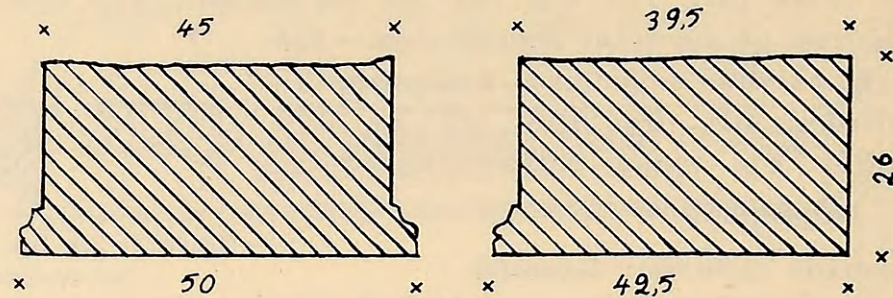
Εἰκ. 16 (ἀρ. 60). Τομή κατὰ μήκος καὶ ἐγκαρσία.
