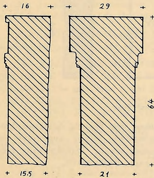
Εἰκ. 40 (ἀρ. 118). Τομὴ κατὰ κρόταφον καὶ ἐγκαρσία.
