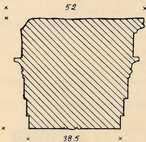
Εἰκ. 8 (ἀρ. 27). Τομὴ ἐπιστυλίου.
