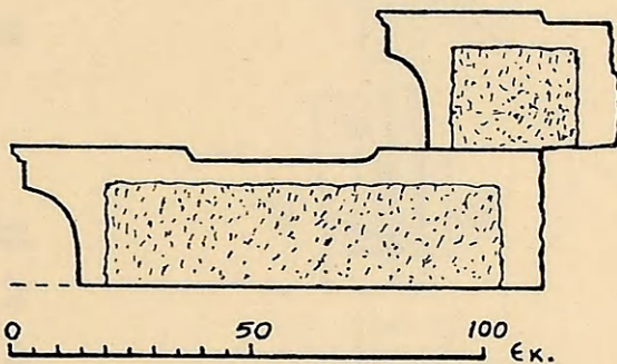
Εἰκ. 22. (IG XII 2, 278 add.) τομὴ ἐδωλίου τοῦ θεάτρου.
