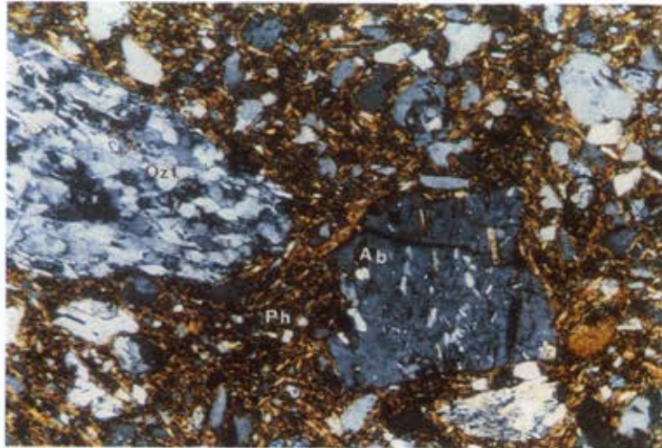
Εικ. 4. Κεραμεικό no 5-Γ, +Nicols X65. Qzt= κλάστες χαλαζίτη, Ab= Άλβίτης, Ph= φυλλώδη όρυκτά.
