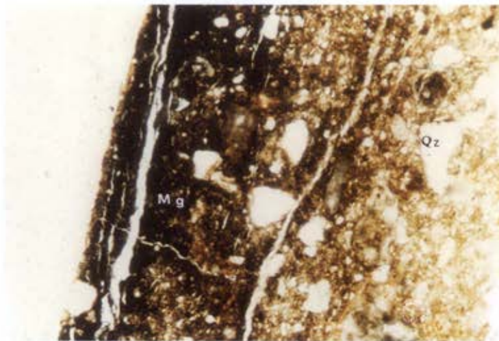
Είκ. 1. Κεραμεικό no 2-A, //Nicols X65. Qz= χαλαζίας, Mg= μαγνητίτης.
