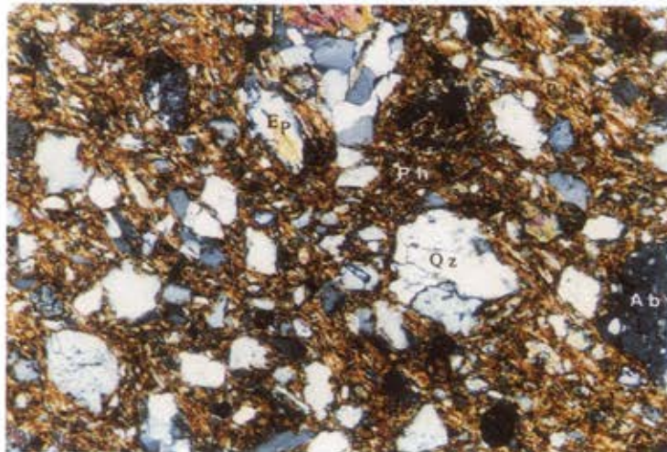
Εικ. 5. Κεραμεικό no 5-Γ, +Nicols X65. Ep= επίδοτο, Qz= χαλαζίας, Ab= Άλβίτης, Ph= φυλλώδη όρυκτά.
