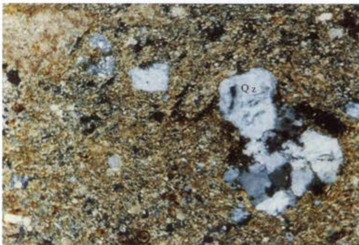
Είκ. 2. Κεραμεικό no 2-A, +Nicols X65. Qz= χαλαζίας.
