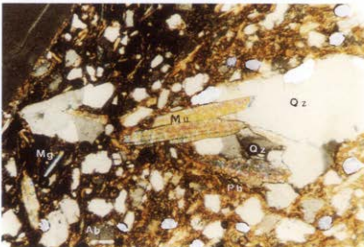
Είκ. 3. Κεραμεικό no 2-B, +Nicols X65. Mg= μαγνητίτης, Qz= άστριοι, Mu= μοσχοβίτης, Ph= φυλλώδη όρυκτά, Ab= άλβίτης.
