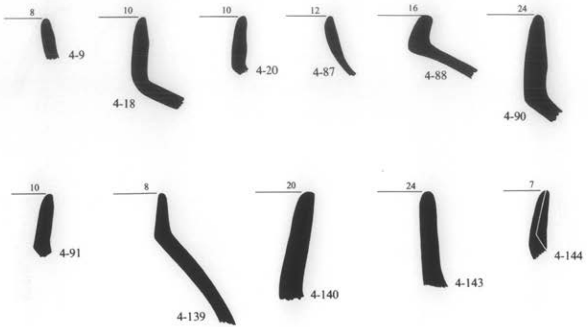
Σχ. 23. Λαιμοί.
